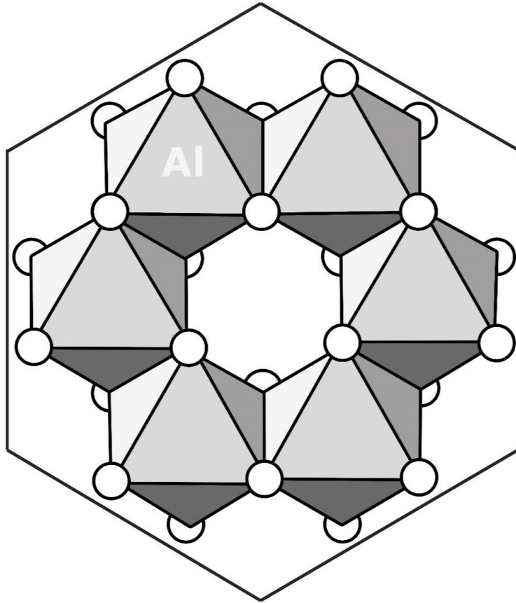
Estructura cristalina simplificada del corindón.
